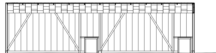
CORTE TRANSVERSAL G-G'
