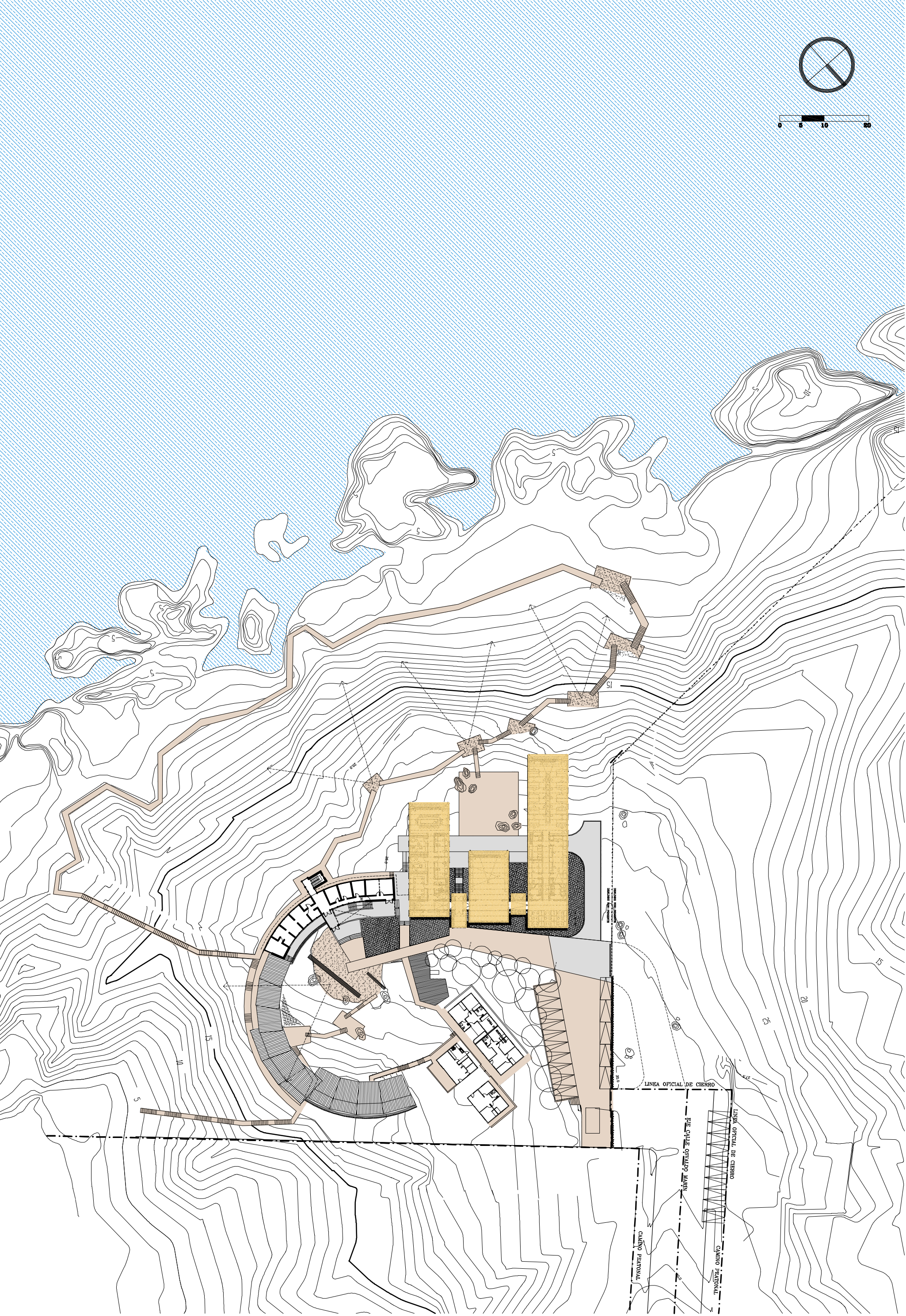
PLANTA DE EMPLAZAMIENTO ESC. 1:750
